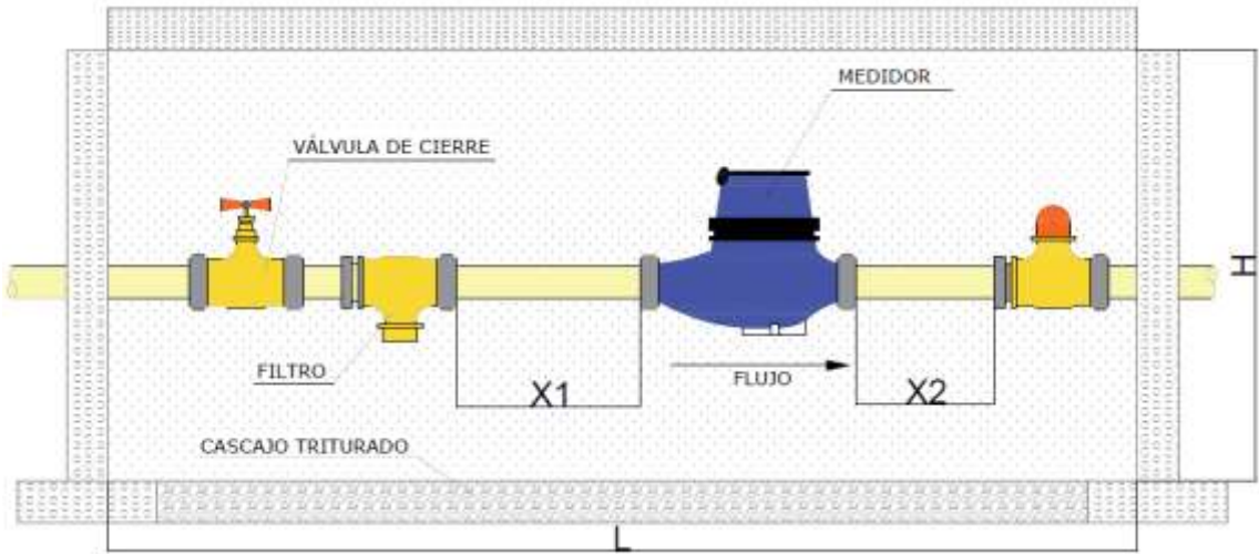
Figura 1. Montaje estación de medición.
